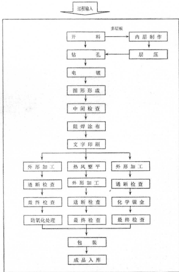
制造工艺流程图
